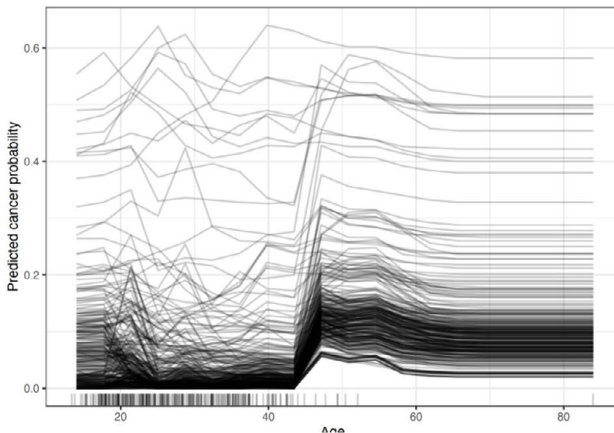
Figura 14. Explicabilitat ICE [24].
