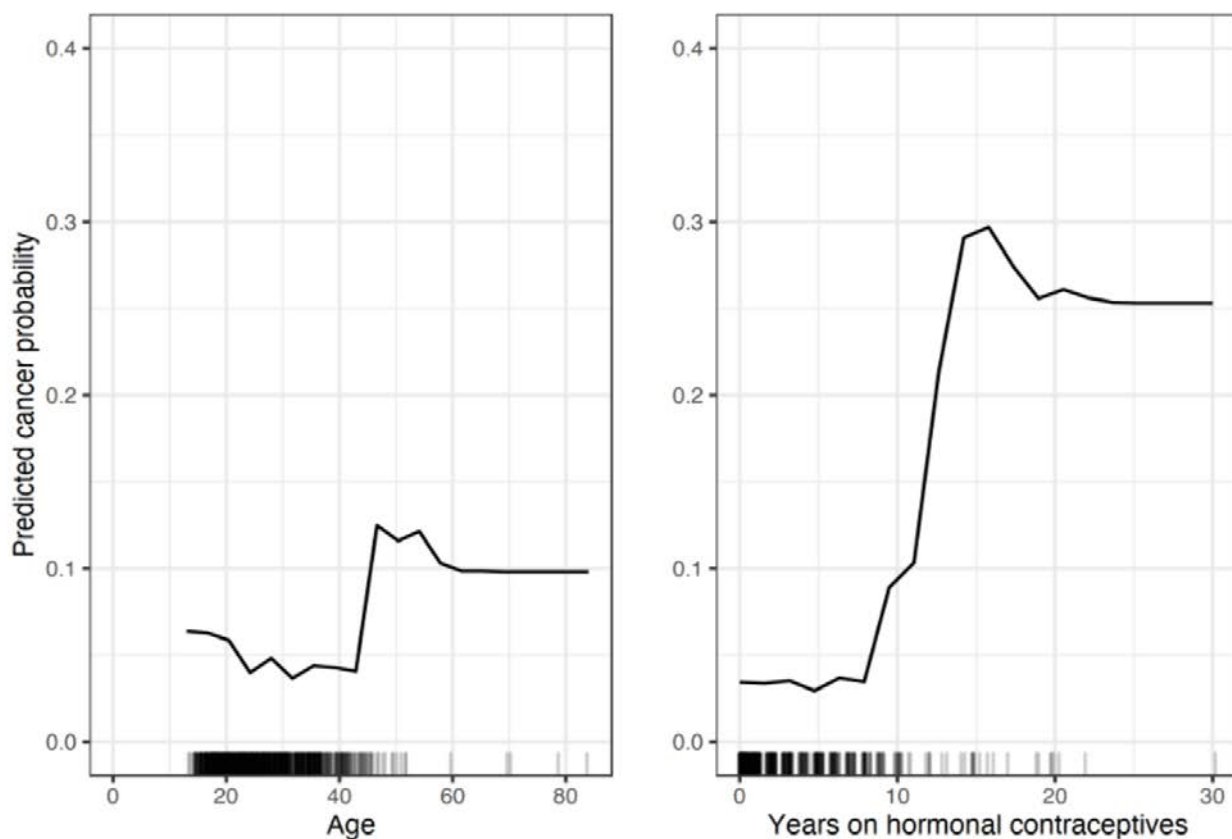
Figura 12. Explicabilitat PDP [23].
