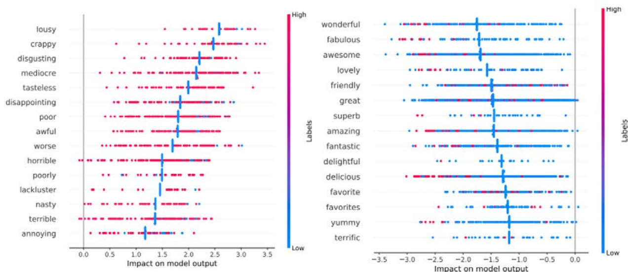
Figura 27. Diagrama d'unicaràcters [32].
