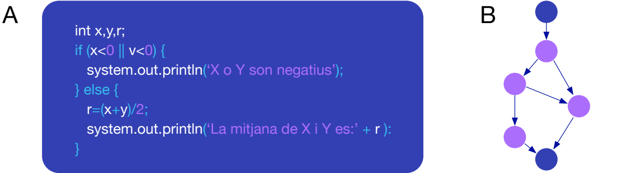
Figura 7. Exemple de càlcul de la Complexitat Ciclomàtica. A: fragment de codi a analitzar; B: esquema de nodes i arestes representatiu de l'execució del fragment de codi de la figura 7A. Els nodes blaus, representen l'entrada i la sortida de l'execució, els taronges les condicions, i les arestes les rutes d'execució.
